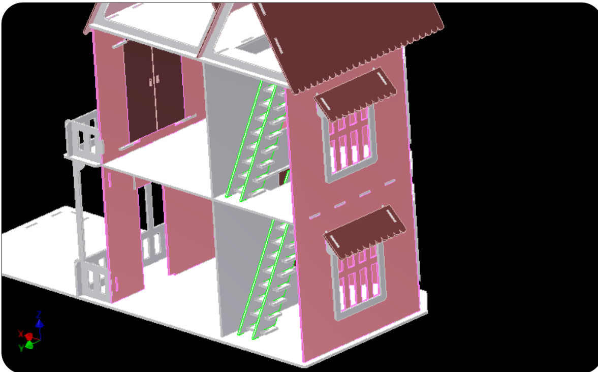
MONTAGEM ESCADA
